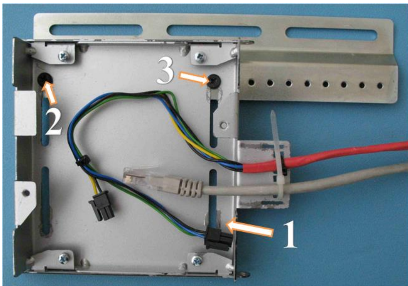
Рисунок 3.2.1 Установка кронштейна платформы КИА
