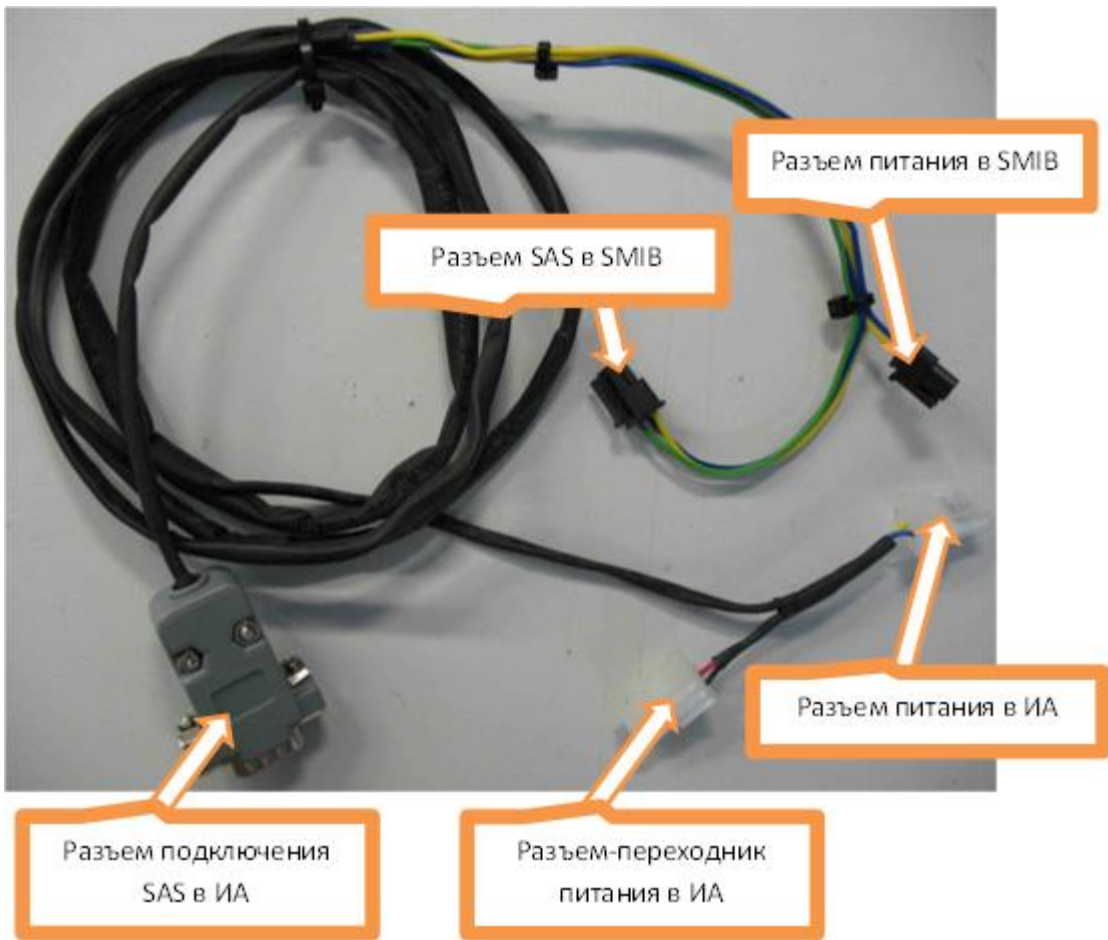
Рисунок 3.4.3 – Кабель соединительный DLV 09-02
