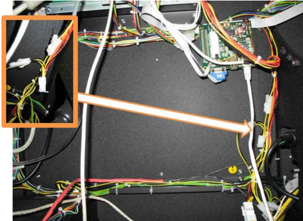
Рисунок 3.4.1 – Подключение питания КИА
