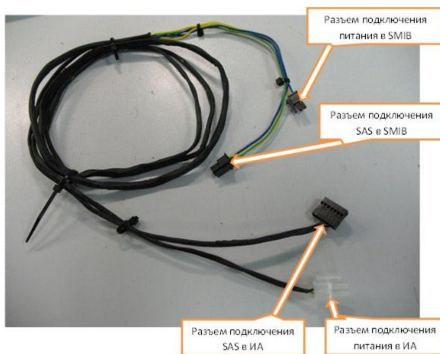
Рисунок 3.4.2 – Кабель соединительный Nov 10-04
