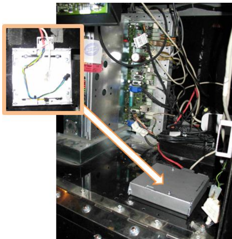
Рисунок 3.1.1 Месторасположение КИА (фронтальный вид ИА)
