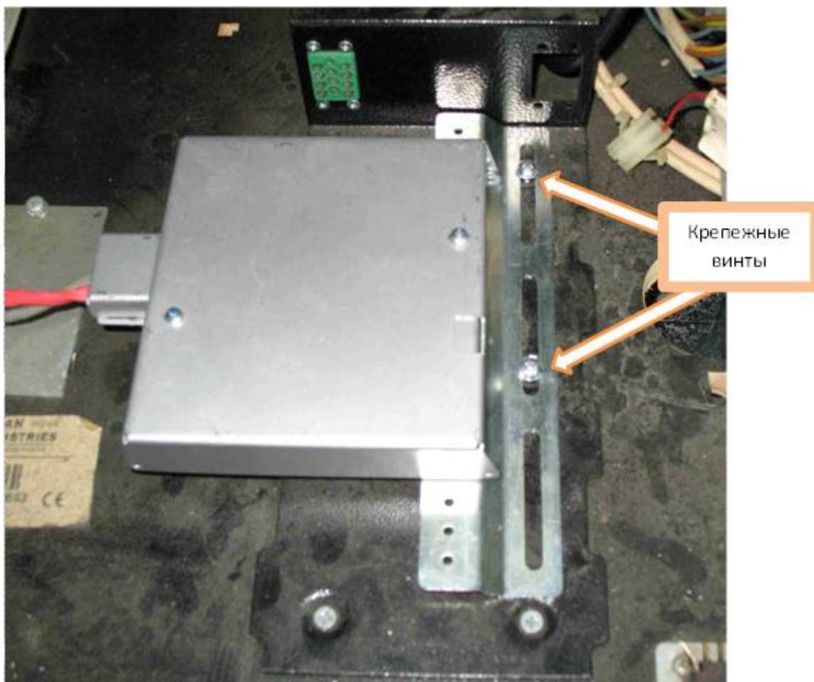
Рисунок 3.3.1 – Закреплённый КИА в ИА
