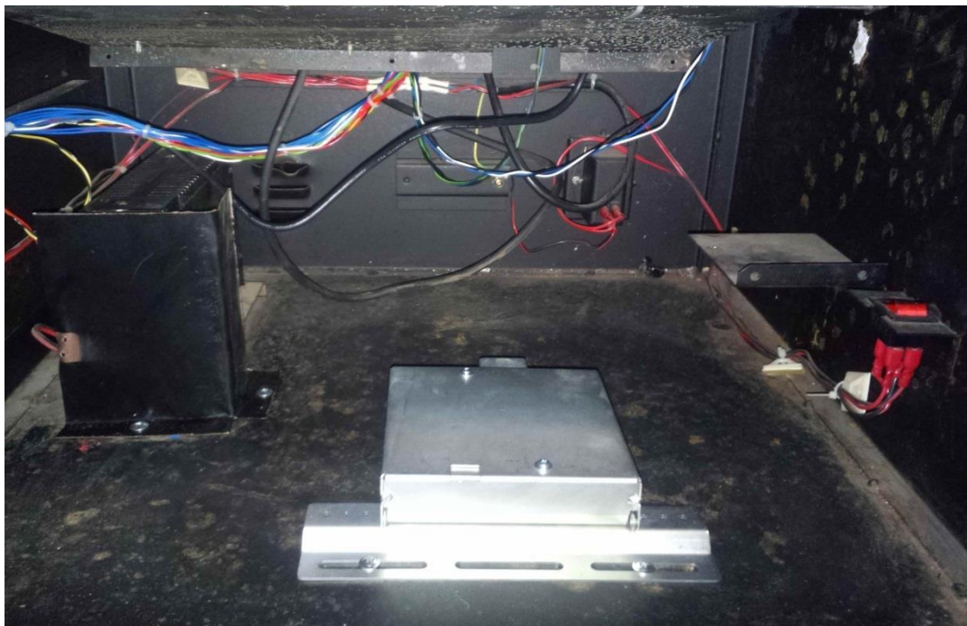
Рисунок 3.1.1 Месторасположение КИА (фронтальный вид ИА)
