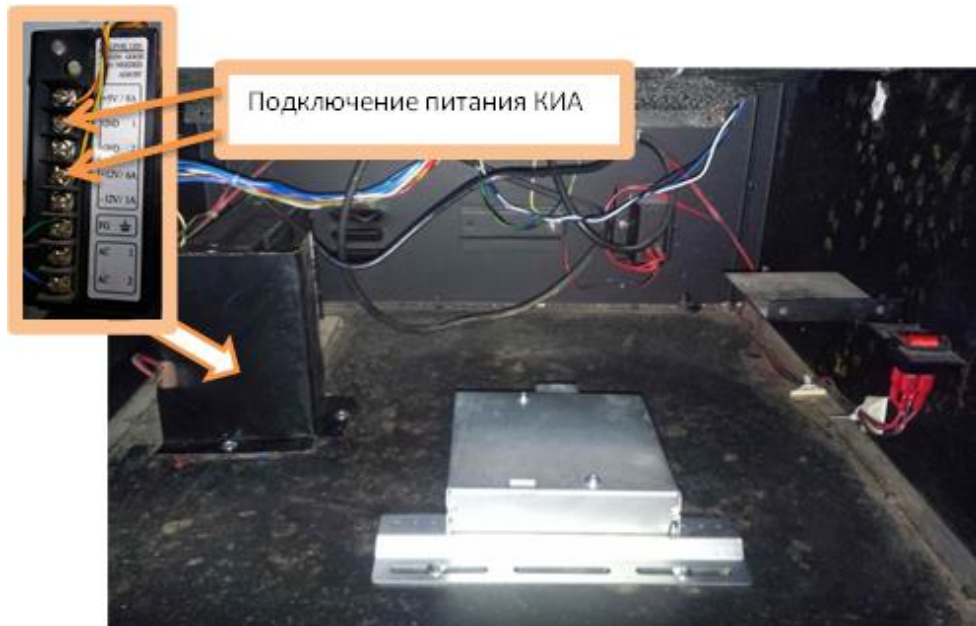
Рисунок 3.4.2 – Подключение питания КИА
