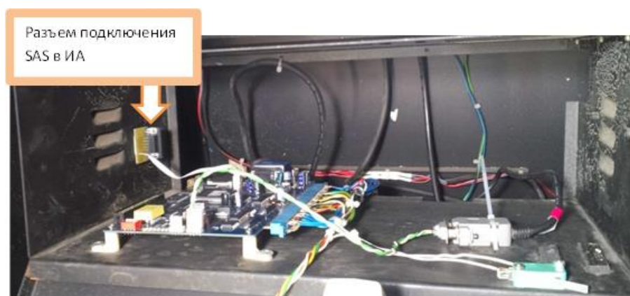
Рисунок 3.4.1 – Переходная плата ИА
