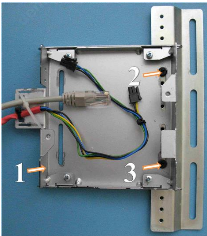
Рисунок 3.2.1 Установка кронштейна платформы КИА
