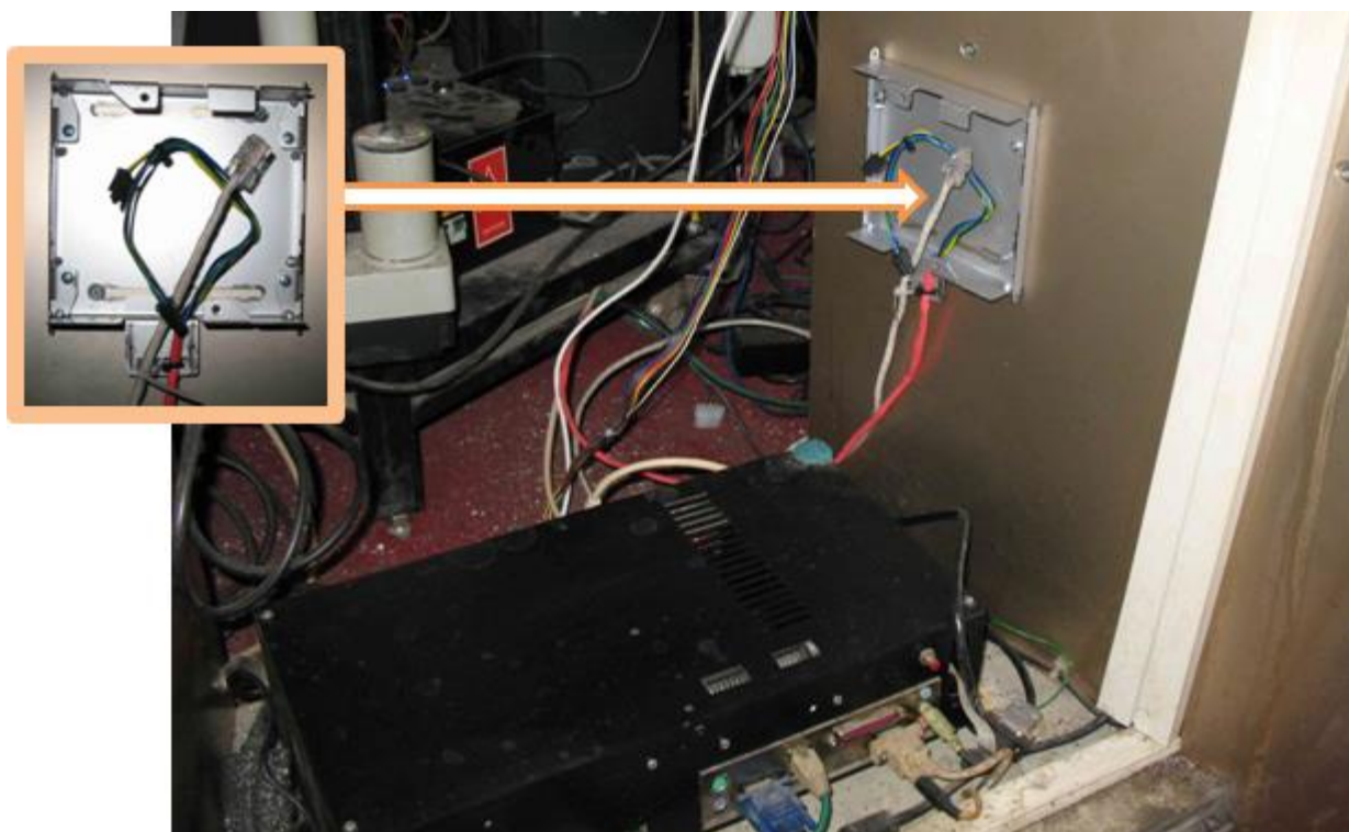
Рисунок 3.1.1 Месторасположение КИА (фронтальный вид ИА)
