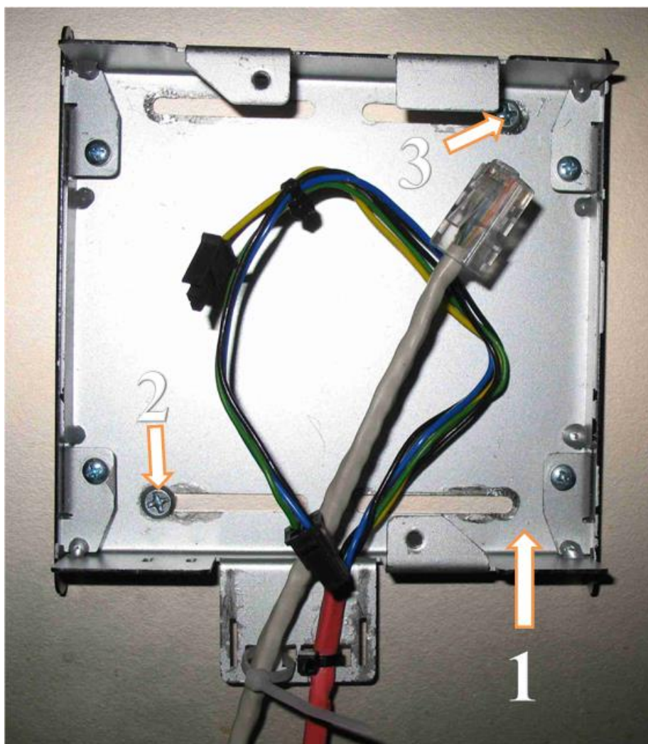
Рисунок 3.3.1 Крепление КИА
