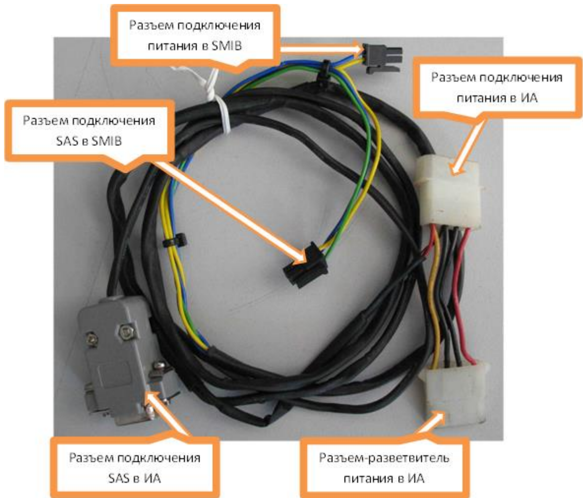
Рисунок 3.4.2 – Кабель соединительный RuI 09-04
